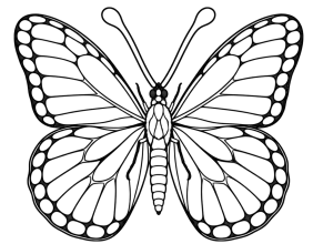
オオカバマダラ
