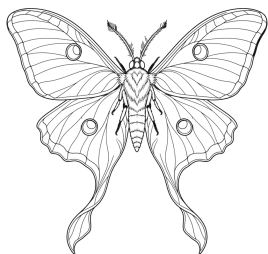
アメリカオオミズアオ
