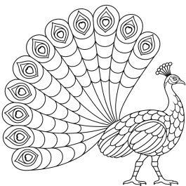
インドクジャク
