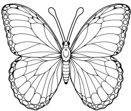
モルフォチョウ
