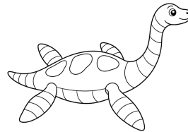
Plesiosaur
