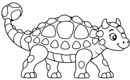
Ankylosaurus
