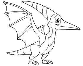
Pteranodon
