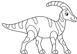
Parasaurolophus
