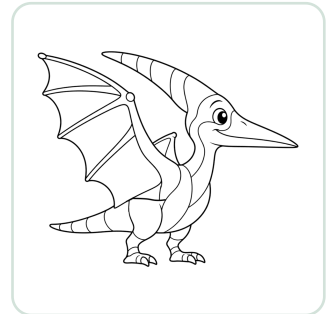
Pteranodonte
